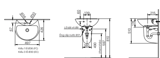
L-285V (EC/FC) | L-288VC
