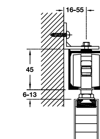
Wall installation with wooden panel Treo tường với nắp che
