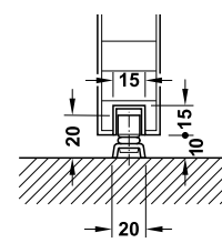
Floor guide with U-shaped guide track in door leaf an floor guide roller Dẫn hướng sàn kèm theo thanh dẫn hướng gắn cửa dạng chữ U và bánh xe
