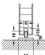
Floor guide without guide track in door leaf Dẫn hướng sàn không gồm thanh dẫn hướng gắn cửa
