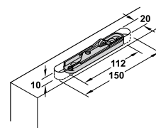
Routing dimension Kích thước khoan cắt
