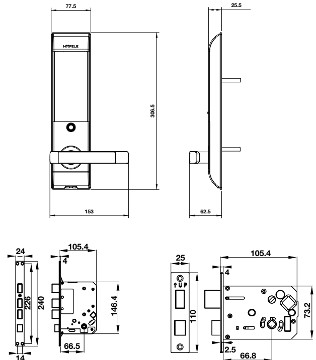
Thân khóa lớn Big mortise
