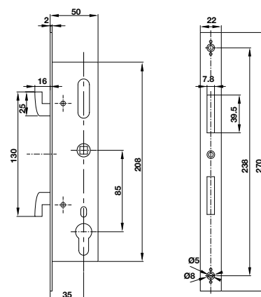
Thân khóa cửa xoay Swing door Mortise
