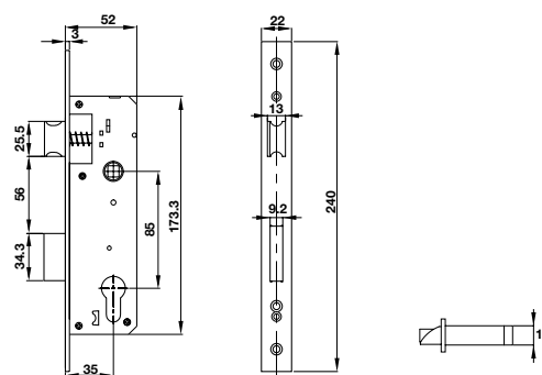
Thân khóa cửa xoay Swing door Mortise
